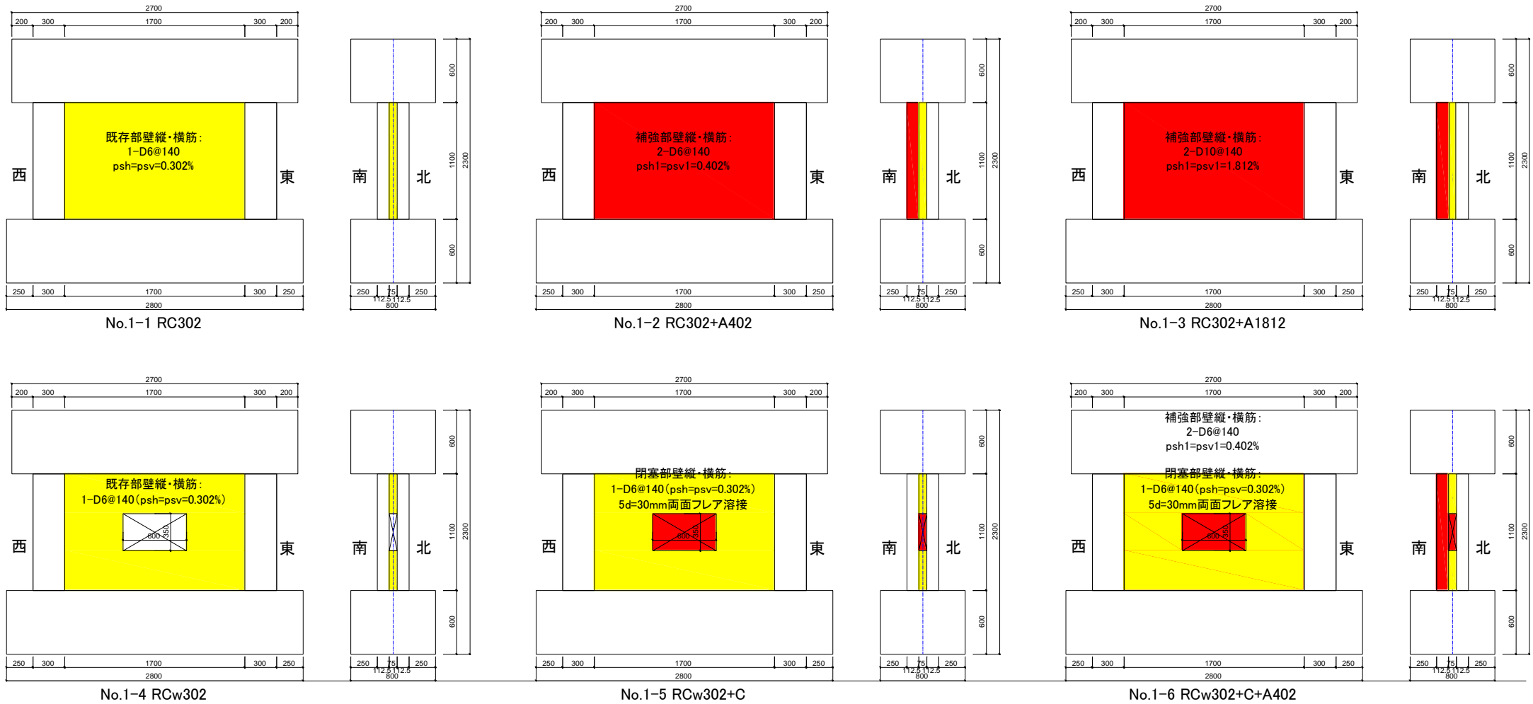
図-3.1.1 試験体形状図
